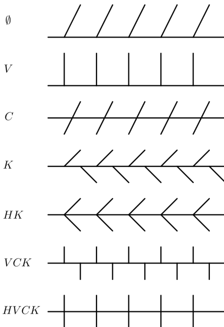
Slika 11: Mogući tipovi frizova
