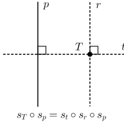
Slika 10: Klizna simetrija prikazana kao kompozicija osne i centralne simetrije
