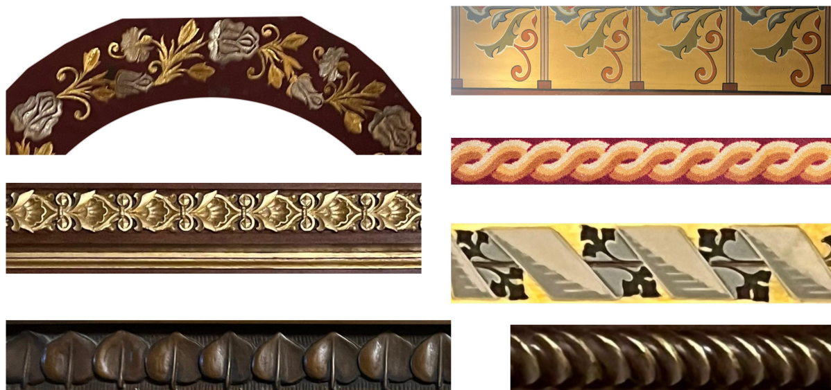
Slika 12: Frizovi tipa Ø (jedine simetrije su translacije)
