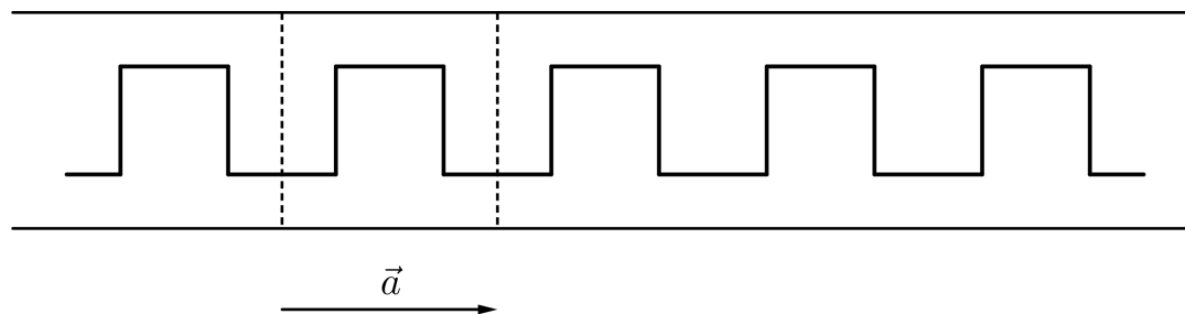
Slika 4: Friz s jednim označenim uzorkom i najkraćim vektorom translacije
