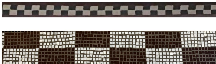
Slika 17: Frizovi tipa VCK . Ako ste razočarani malim brojem primjera ovog tipa frizova u konkatedrali, prošetajte se do obližnje crkve svetog Marka gdje ćete ih na poznatom šarenom krovu uočiti još nekoliko.
