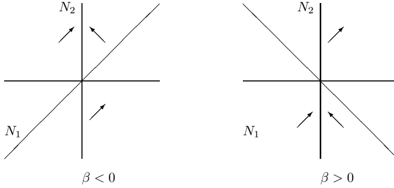
Figure 4 : \delta \neq 0
