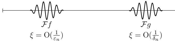
Slika 4. Fourierov prostor s dvije različite skale.
