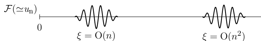
Slika 1. Očekivana skala u Fourierovom prostoru.
